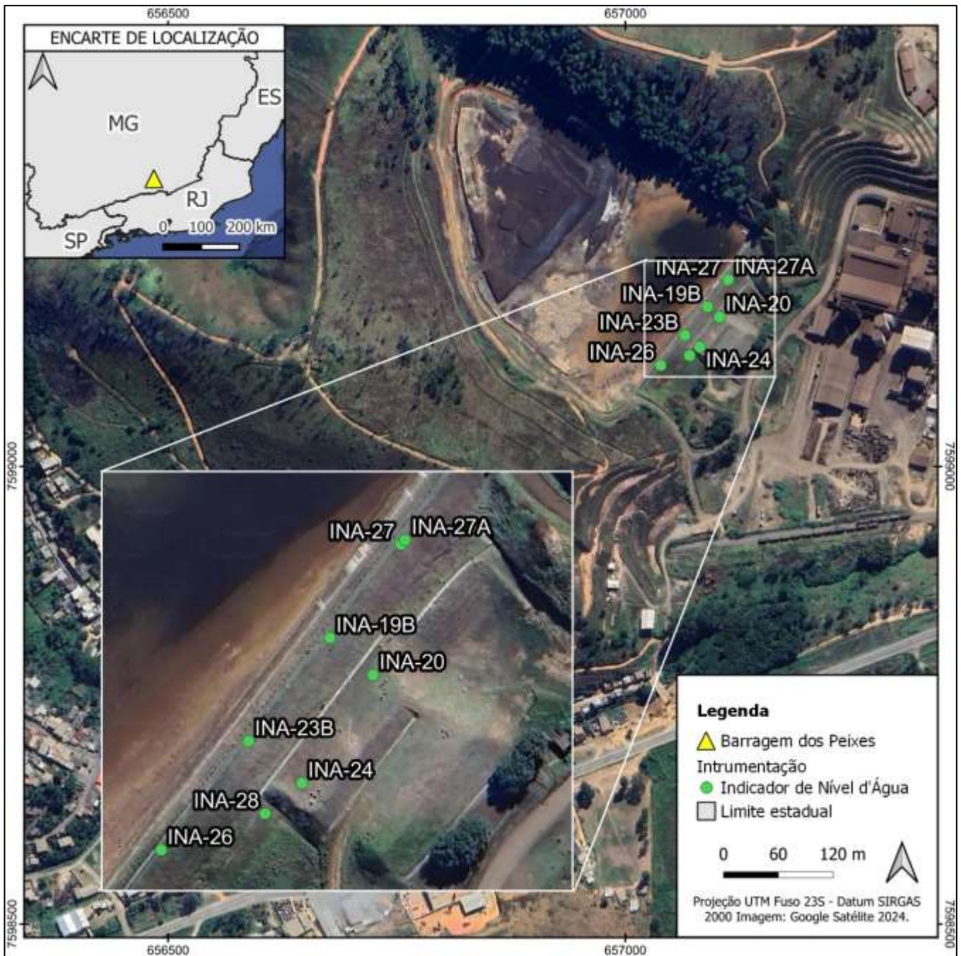
Figura 5.2 - Instrumentação da Barragem dos Peixes – Indicadores de Nível d'Água – Cisalhamento.
