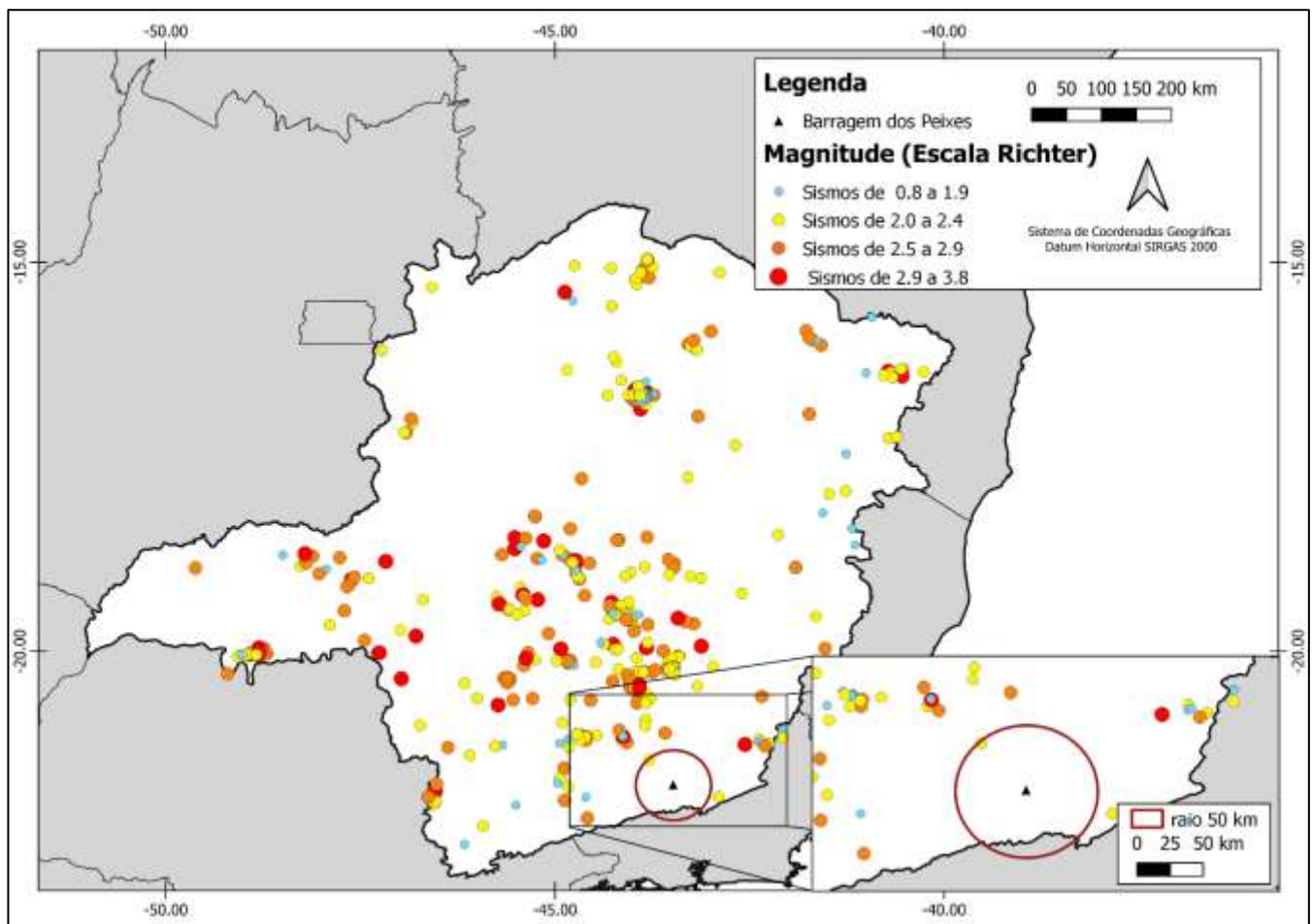
Figura 4.14 - Atividades sísmicas em Minas Gerais entre 1980 e 2024.
