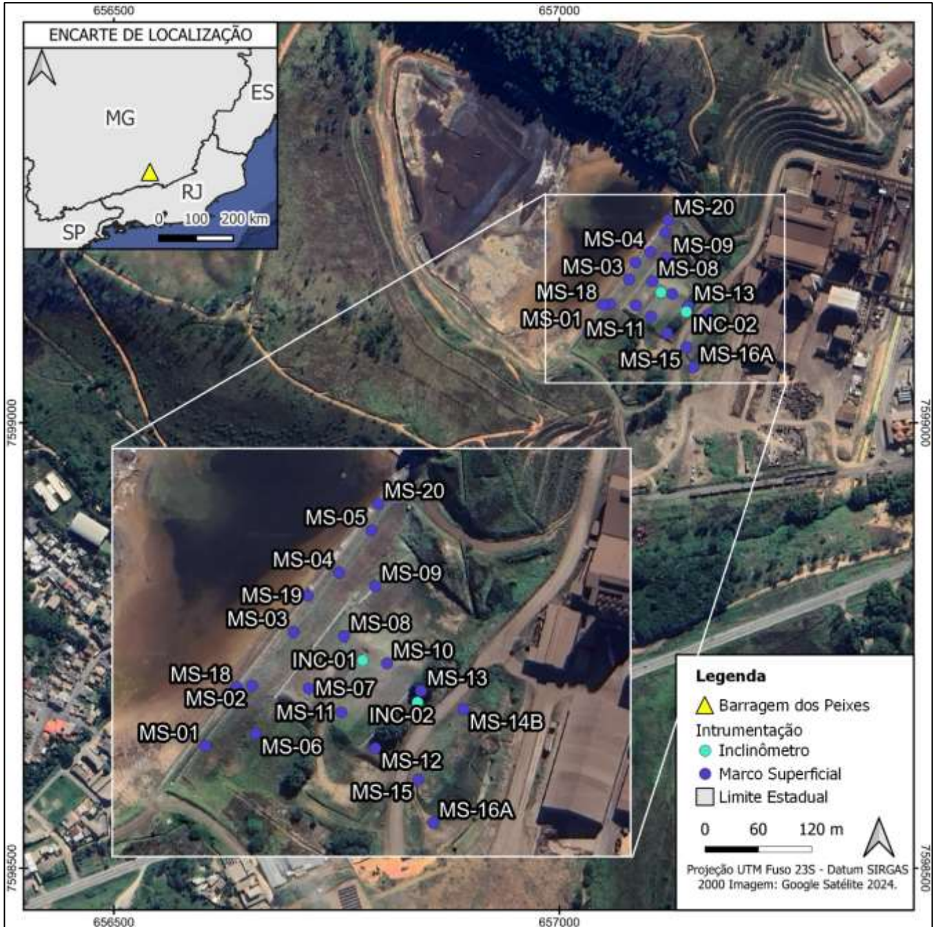
Figura 5.3 - Instrumentação da Barragem dos Peixes – Inclinômetros e Marcos Superficiais.
