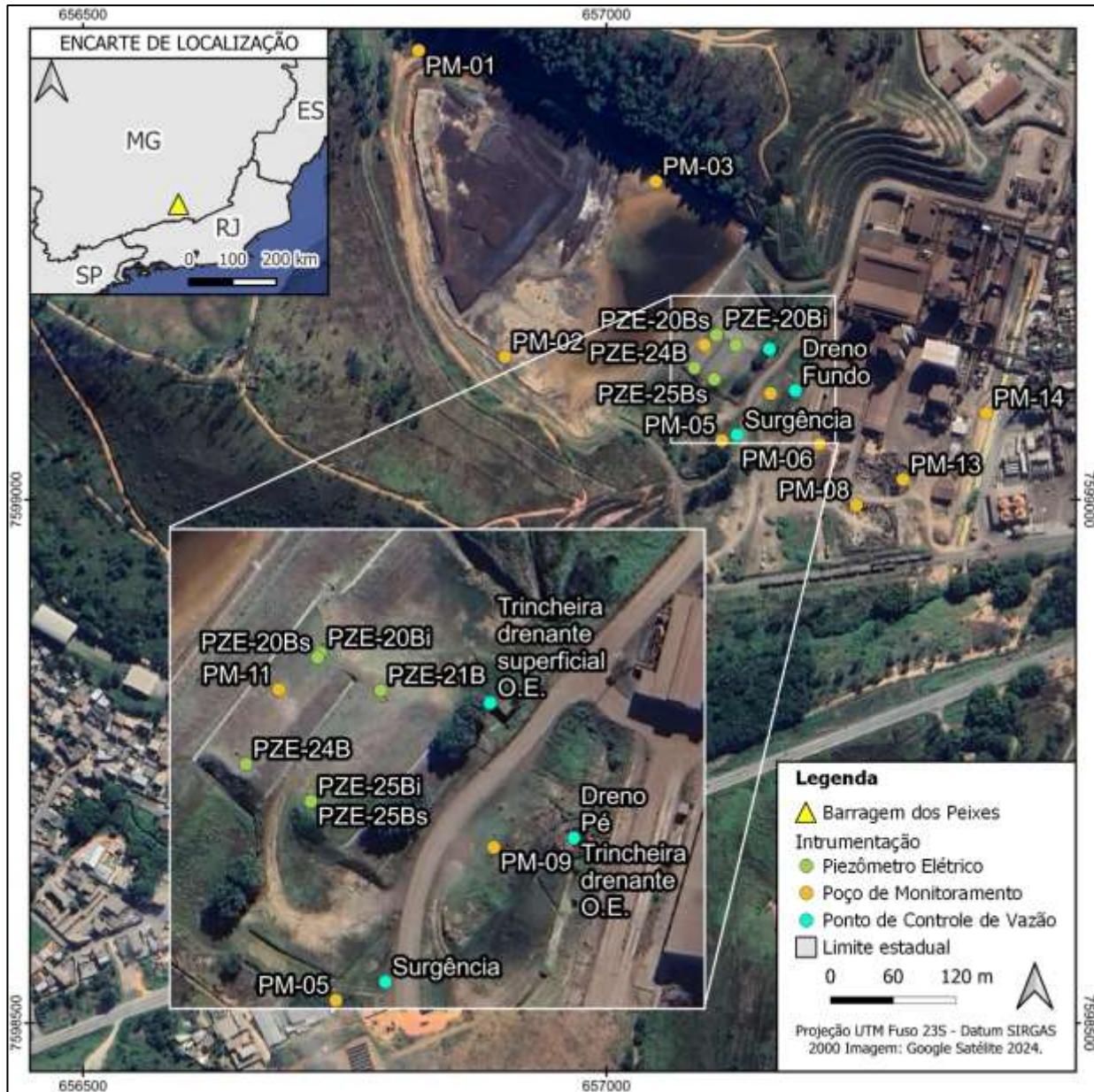
Figura 5.1 - Instrumentação da Barragem dos Peixes – Piezômetros, Medidores de vazão e Poços de Monitoramento– Piping.
